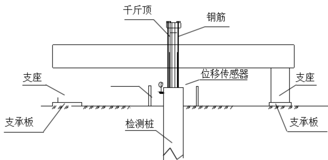
试验装置示意图
